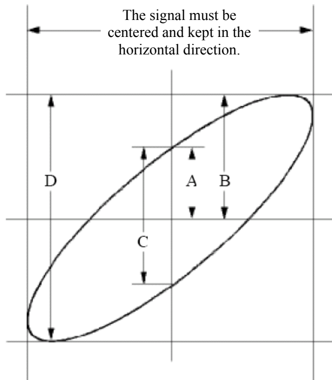
Fig.6-6 Lissajous Graph
